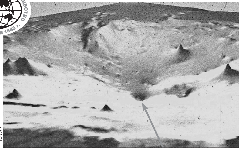
3D-модель дна Чеко - оно имеет необычную форму, больше похожую на кратер. В указанной точке, вероятно, и скрывается осколок космического пришельца.
