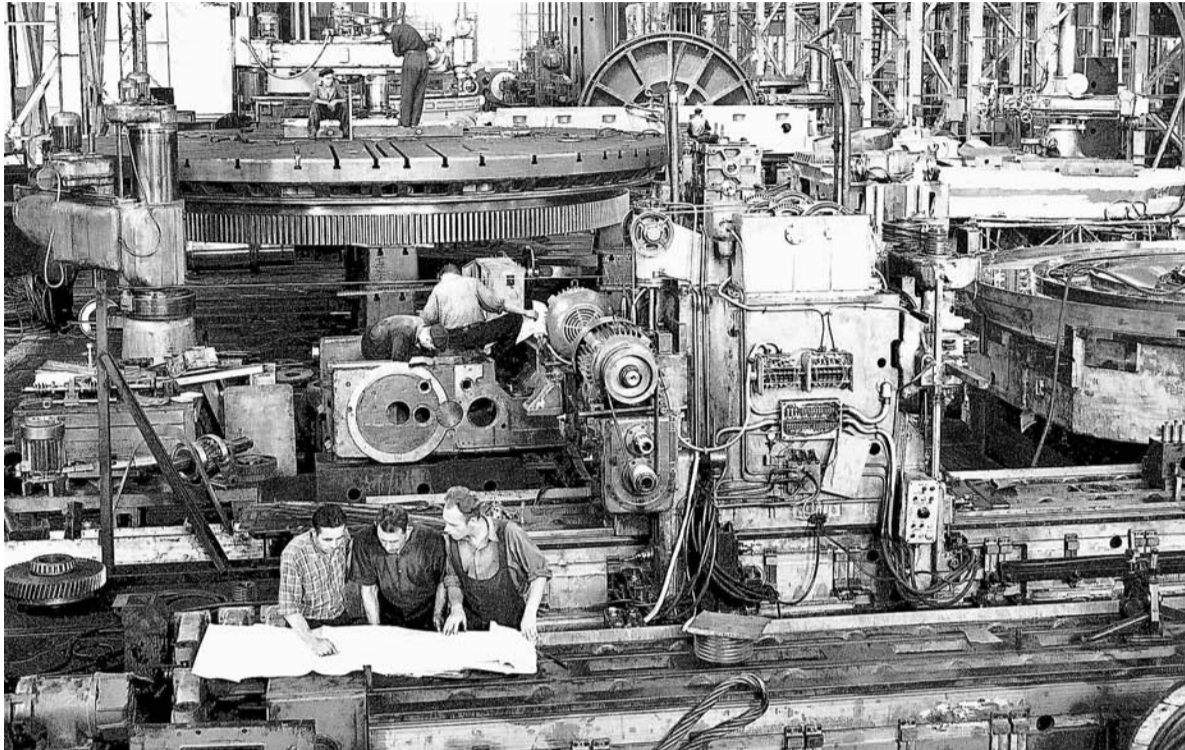
Сборочный цех Коломенского завода тяжёлых станков, 1959 г. Завод выпускал до 200 тяжёлых металлообрабатывающих станков и 20 мощных прессов в год. Фото РИА Новости
